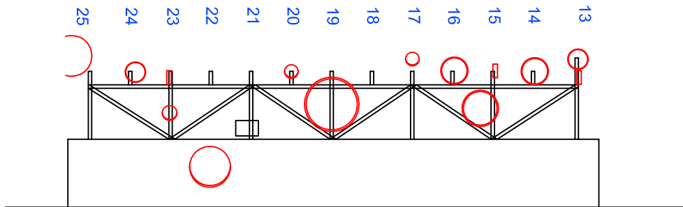
SE Elevation
